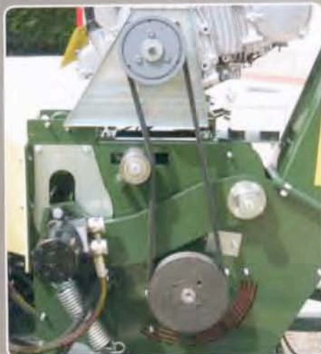
Trasmissione a cinghia con frizione centrifuga per versione motore. Belt transmission with centrifugal clutch for version with gasoline engine Transmission par courroie avec embrayage centrifuge pour version avec moteur à essence Correa de transmisión con embrague centrifugo para version motor de gasolina Kiemenantrieb mit Zentrifugalkupplung für die Ausführung mit Benzinmotor Riemoverbrenging met centrifugaalkoppeling voor de versie met benzienmotor
