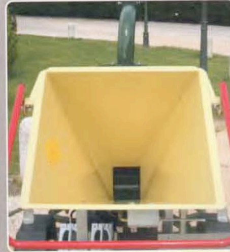
Tramoggia di carico, rullo trascinatore e particolare del maniglione di comando Feeding hopper, feeding roller and detail of the control handle Trémie d'introduction, rouleau ameneur et détails de la poignée de commande Tolva de carga, mando de arrastre, detalles de manubrio de mando Zuführtrichter, Mithemerwelle und Detail des Steuerungshandgriffs Aanvoertrechter, invoerrol, details voor de bedieningshandel
